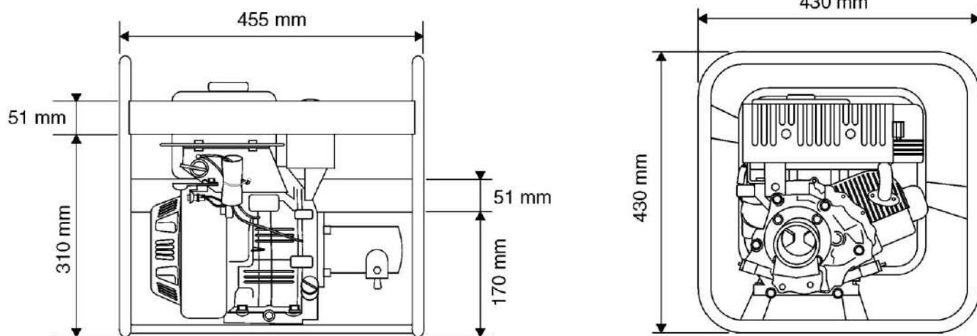
Figura 5. Unidad motriz tipo bastidor
