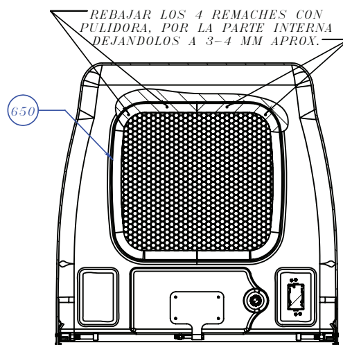
SECCIÓN J-J
