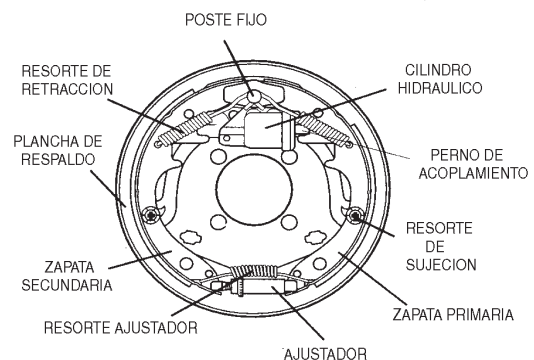
Figura 45. Componentes de los frenos hidráulicos Accionador del freno hidráulico
