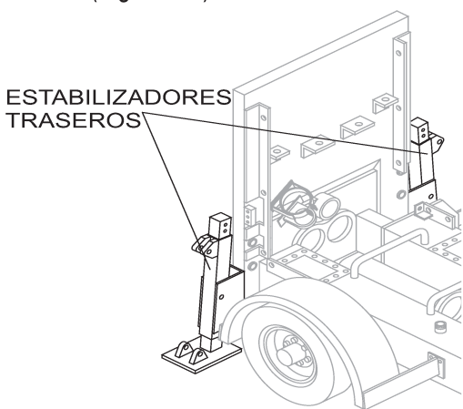
Figura 15. Localizando los estabilizadores traseros
