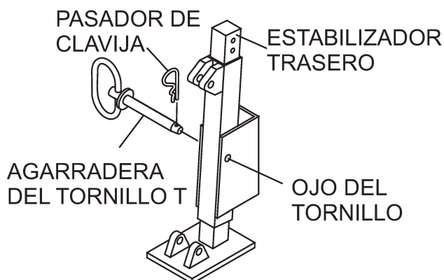
Figura 16. Estabilizador trasero
