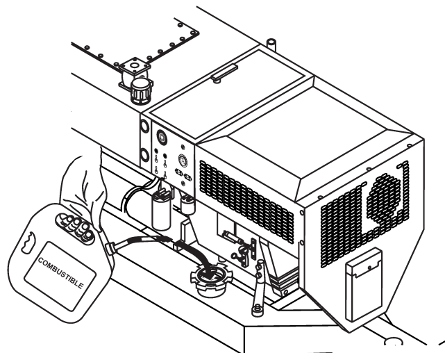
Figura 9. Abasteciendo diesel
